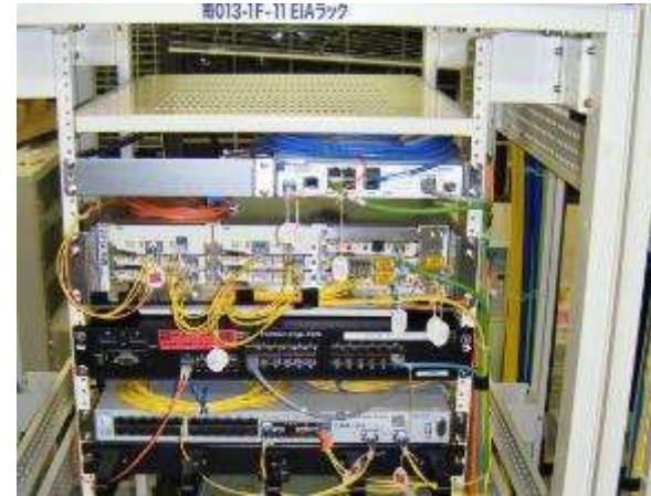
NW 部屋
